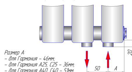
Узел нижнего подключения радиатора Гармония нп
